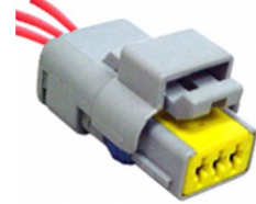
TH-8049 • Sensor temperatura Citroën, Renault, Fiat MTE-4082 3 vias
